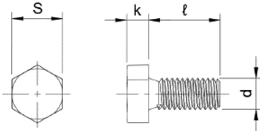
六角ボルト
