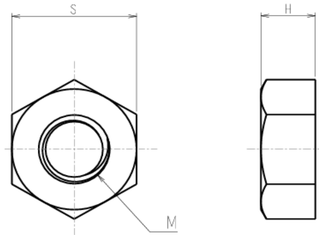
六角ナット
