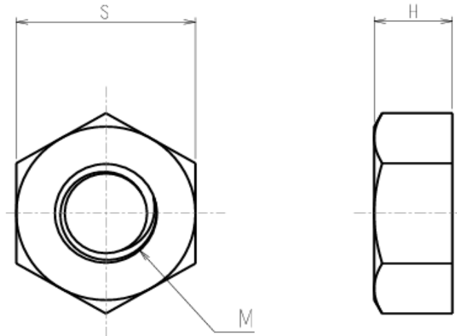
六角ナット
